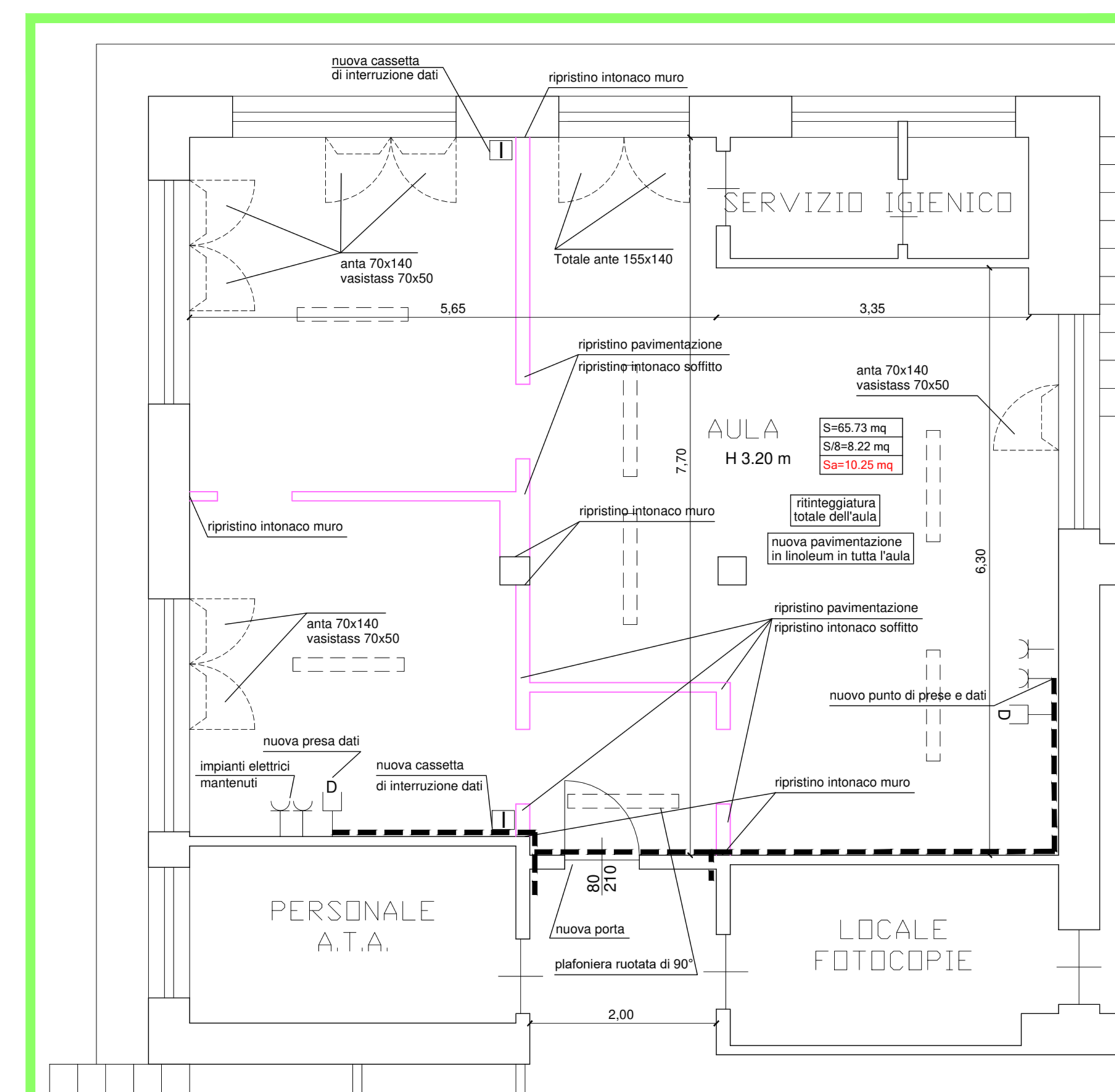
PARTICOLARE 1 - PROGETTO SCALA 1:50
