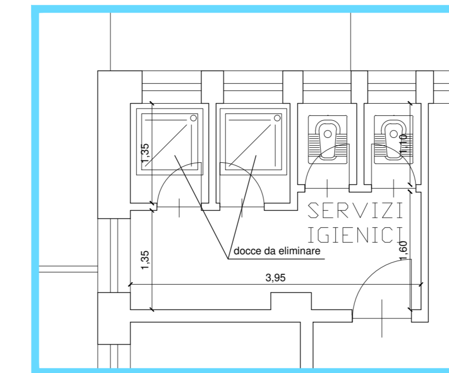
PARTICOLARE 2 - STATO DI FATTO SCALA 1:50
