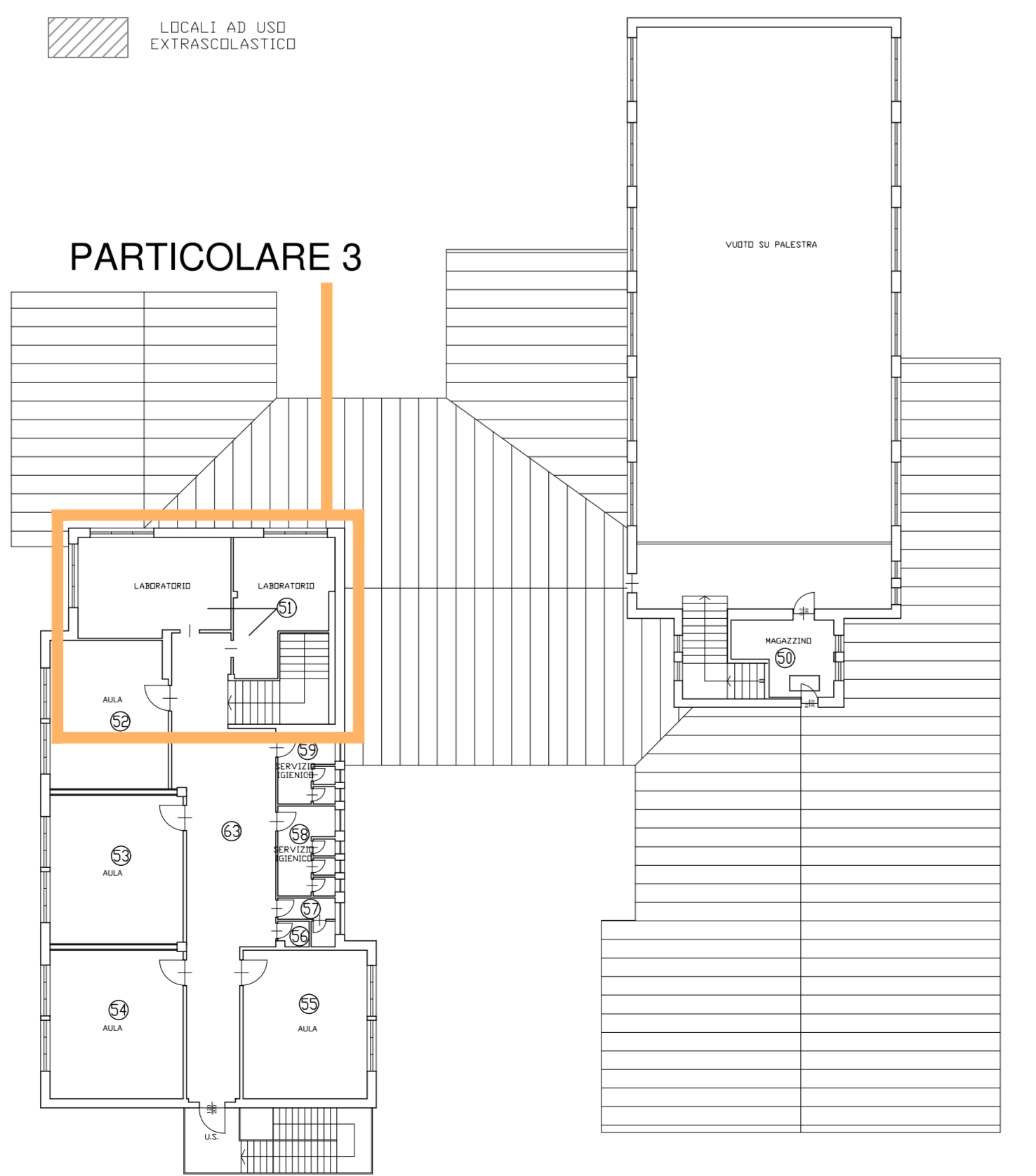
PIANTA PIANO PRIMO SCALA 1:250
