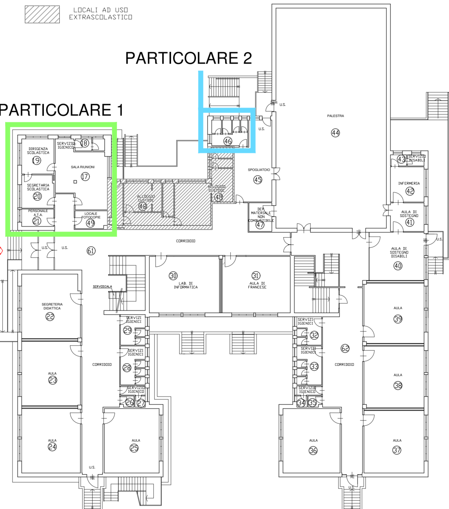
PIANTA PIANO RIALZATO SCALA 1:250
