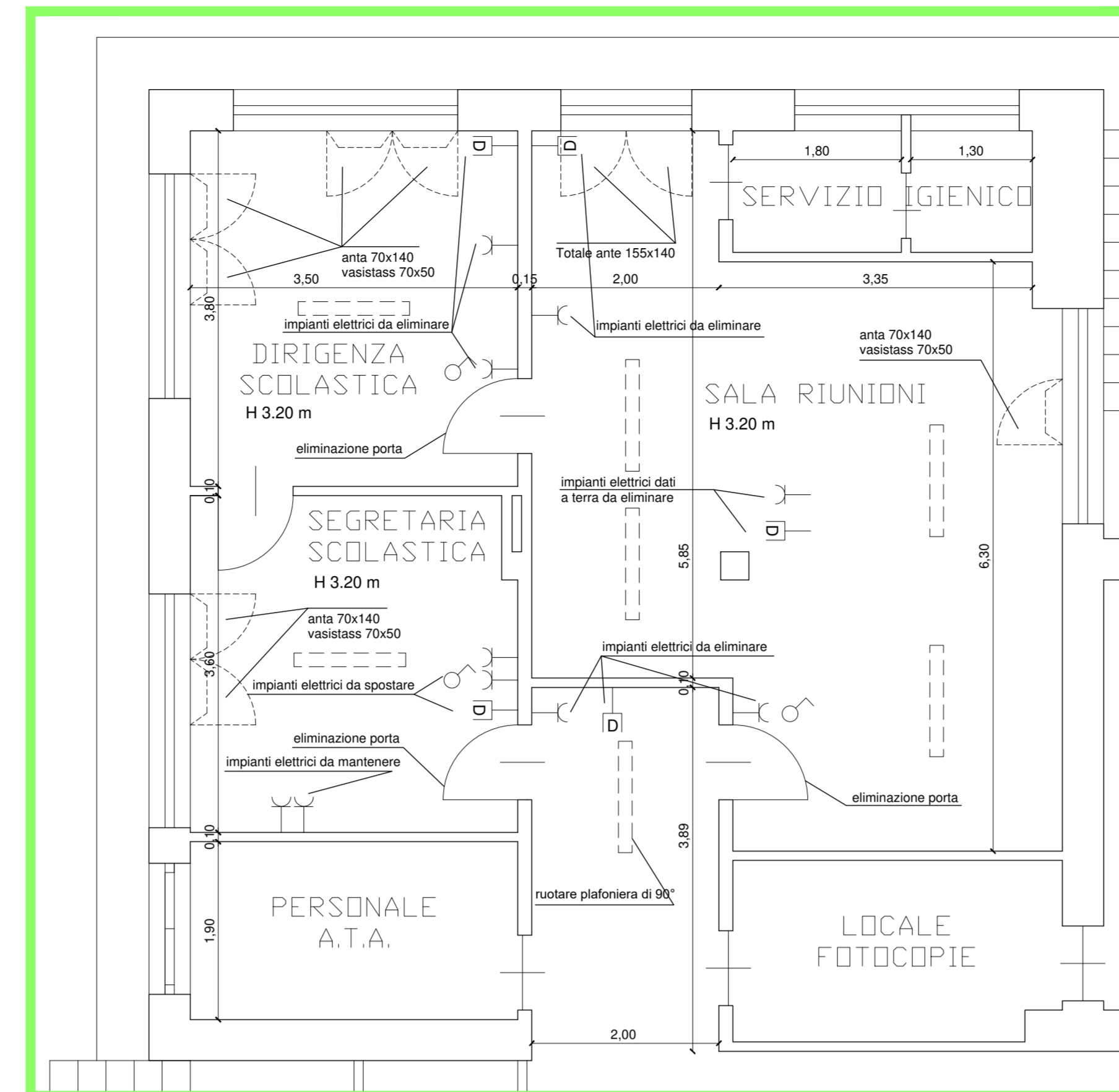
PARTICOLARE 1 - STATO DI FATTO SCALA 1:50
