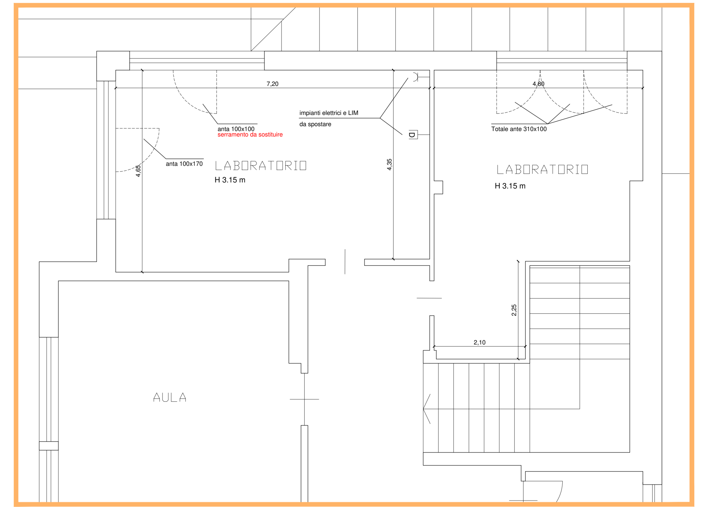
PARTICOLARE 3 - STATO DI FATTO SCALA 1:50
