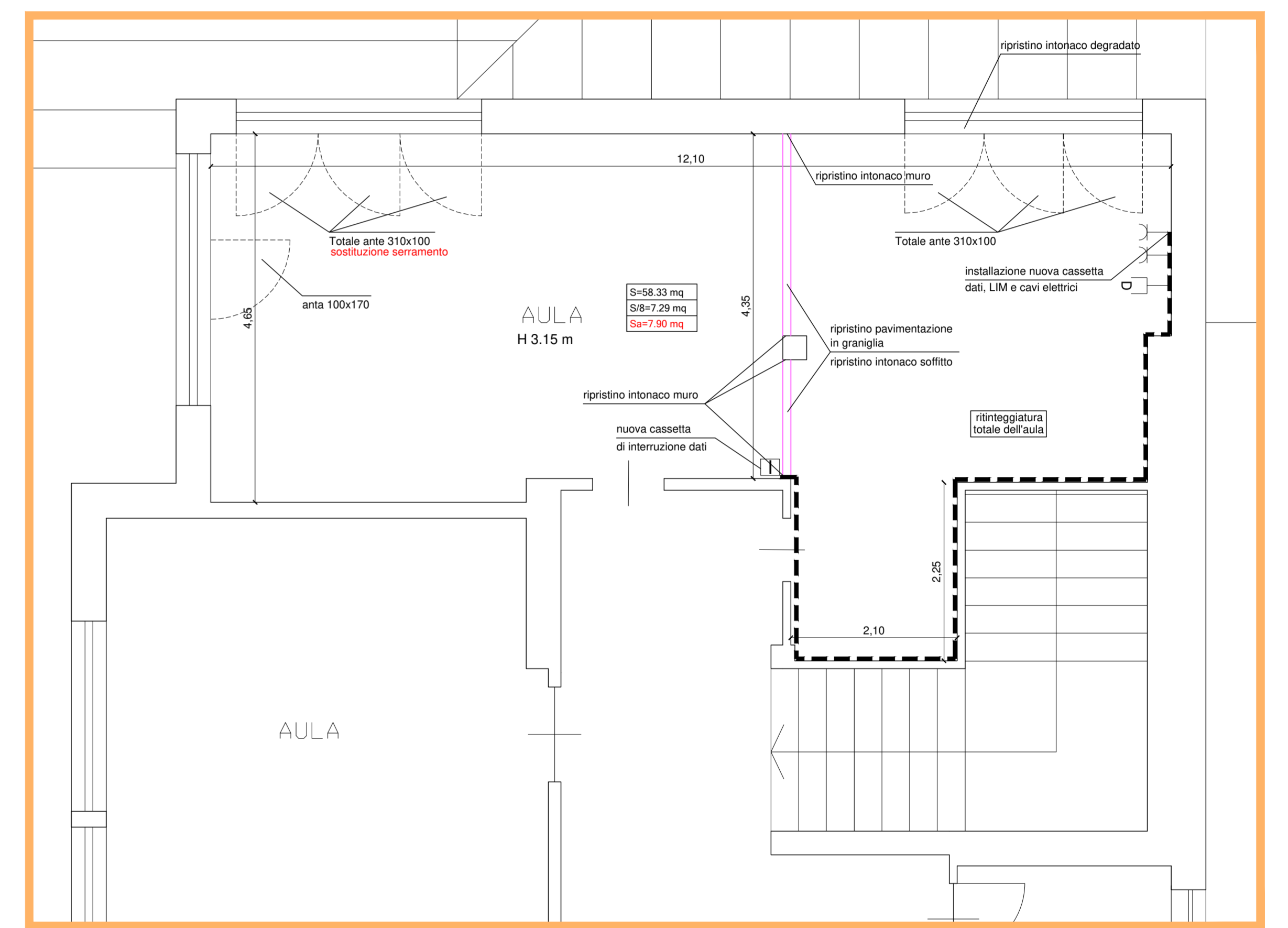
PARTICOLARE 3 - PROGETTO SCALA 1:50
