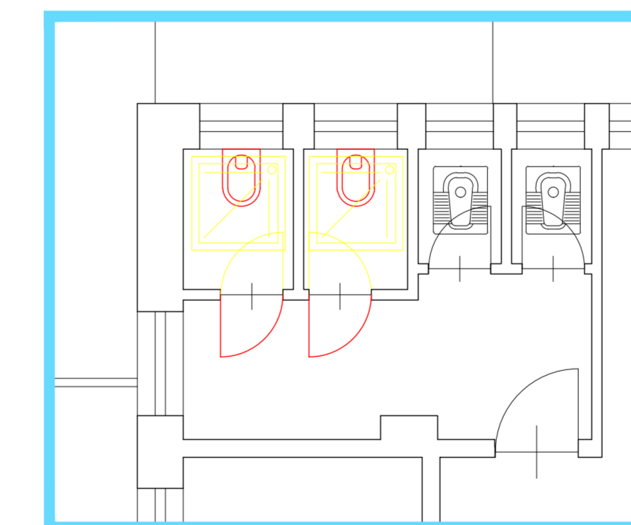
PARTICOLARE 2 - SOVRAPPOSIZIONI SCALA 1:50
