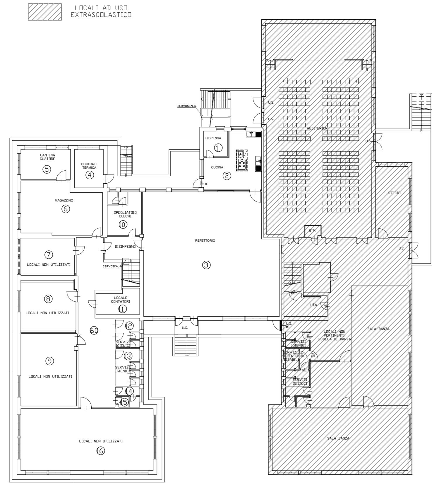
PIANTA PIANO SEMINTERRATO SCALA 1:250
