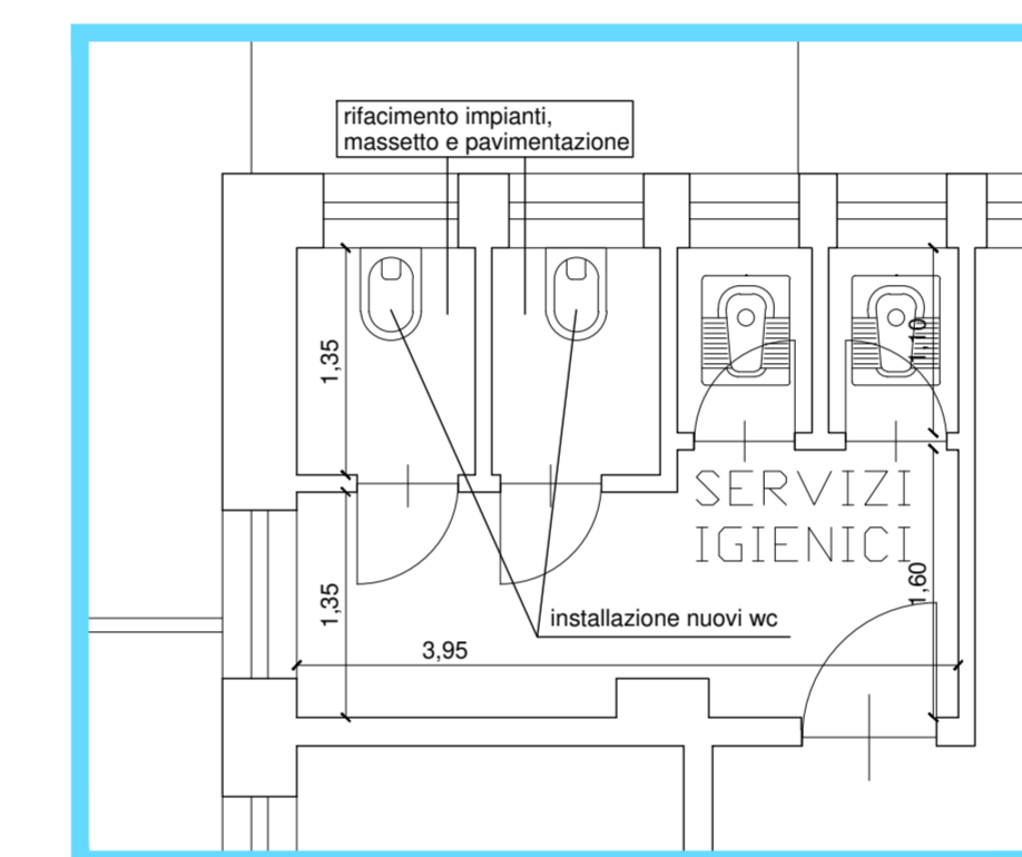
PARTICOLARE 2 - PROGETTO SCALA 1:50
