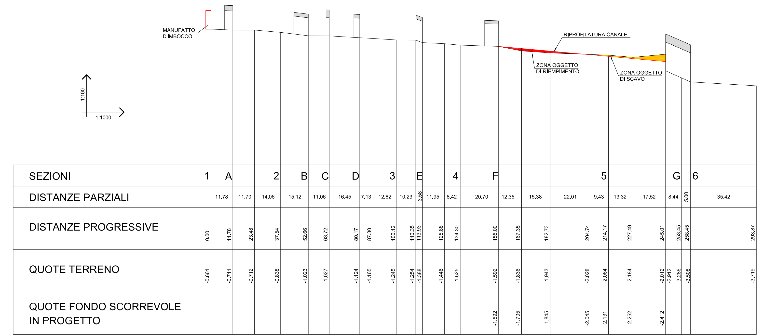
PROFILO LONGITUDINALE CANALE ESISTENTE RIPROFILATURA FONDO CANALE
