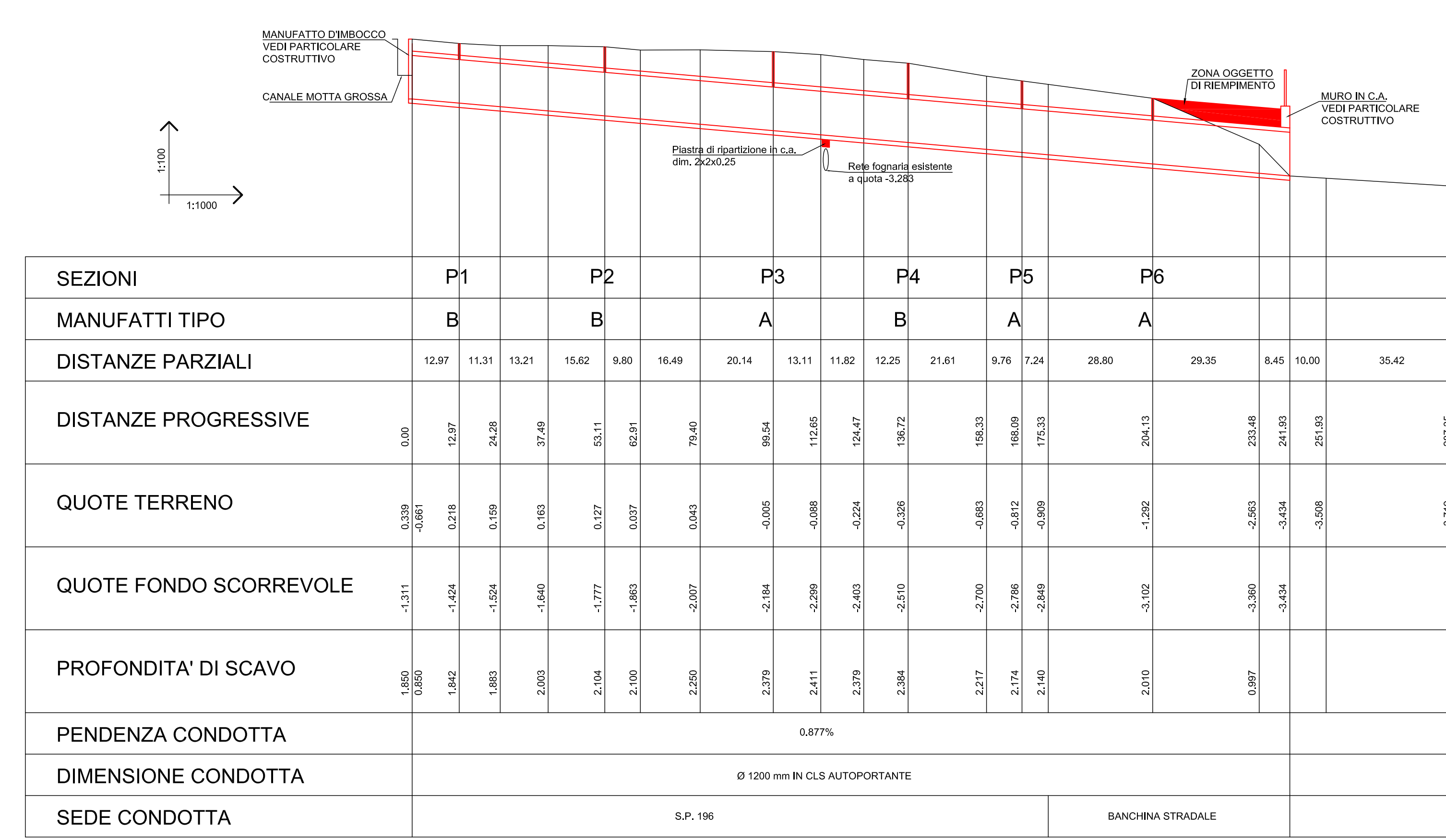
PROFILO LONGITUDINALE CANALE IN PROGETTO
