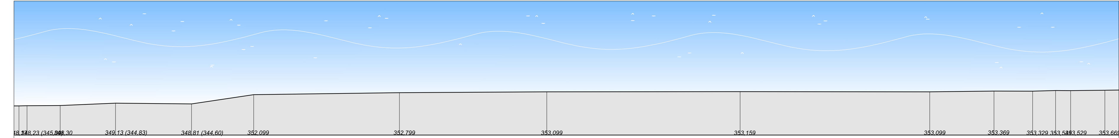
COMUNE DI PINEROLO - Area De 6.1 - Subarea b2 - PROFILO TERRENO ESISTENTE BB'
