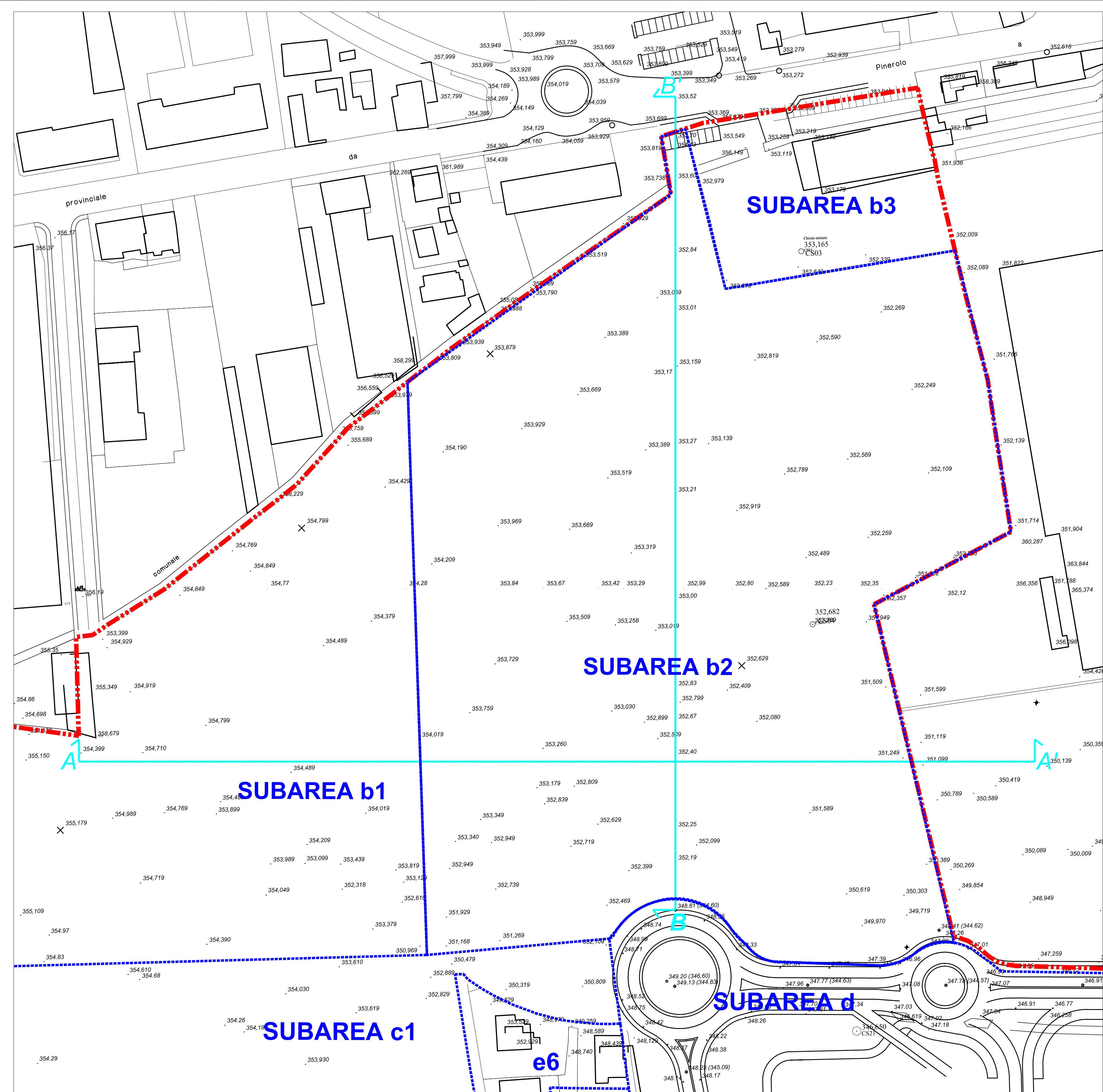
COMUNE DI PINEROLO - Area De 6.1 - Subarea b2 - RILIEVO DELL'AREA
